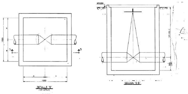
Figura 38 –Detalle de arquetas de conexión de tubería de PCI al edificio de Oficinas y Talleres
