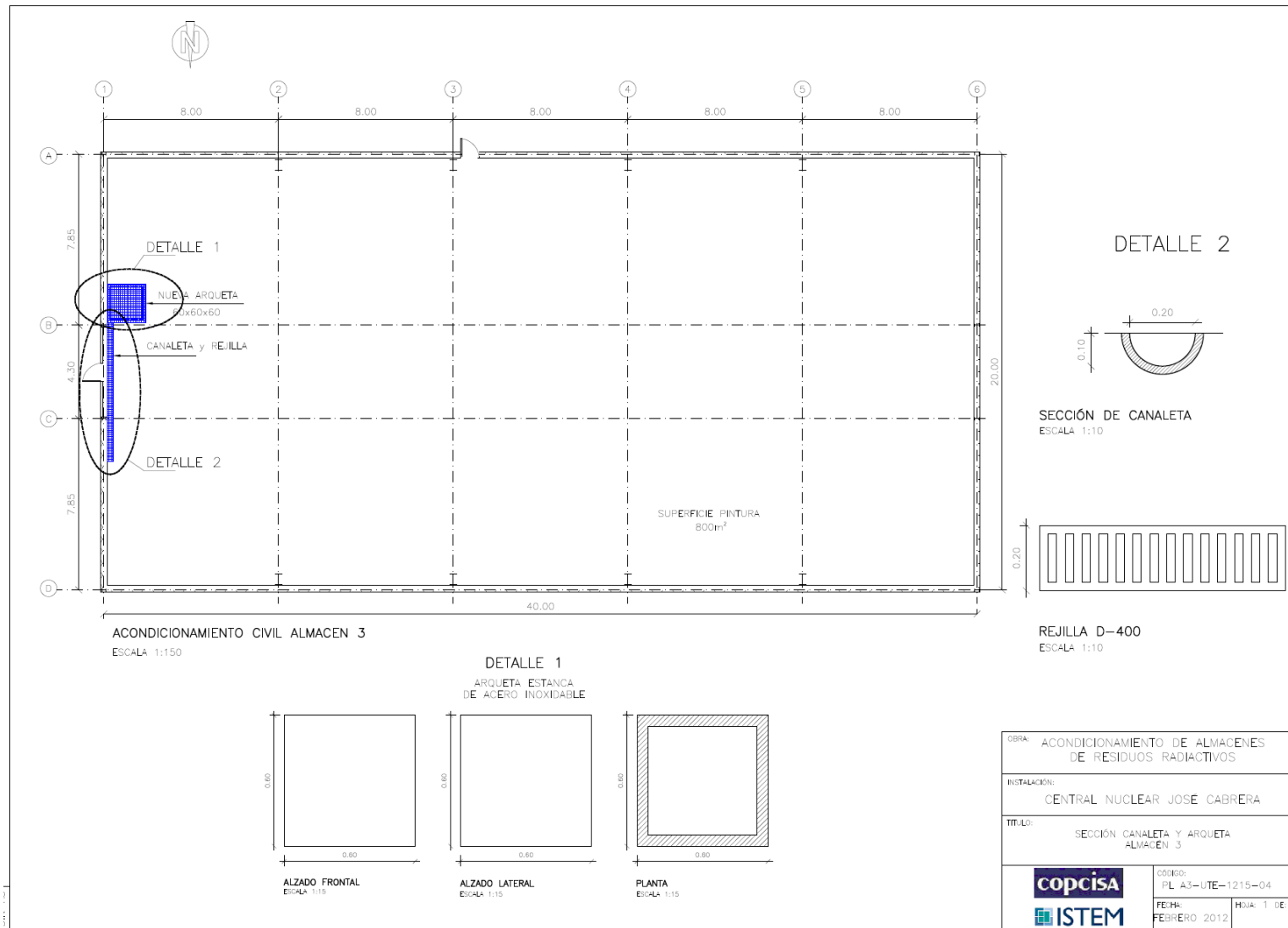
4.- Almacén 3. Planta y detalle arqueta
