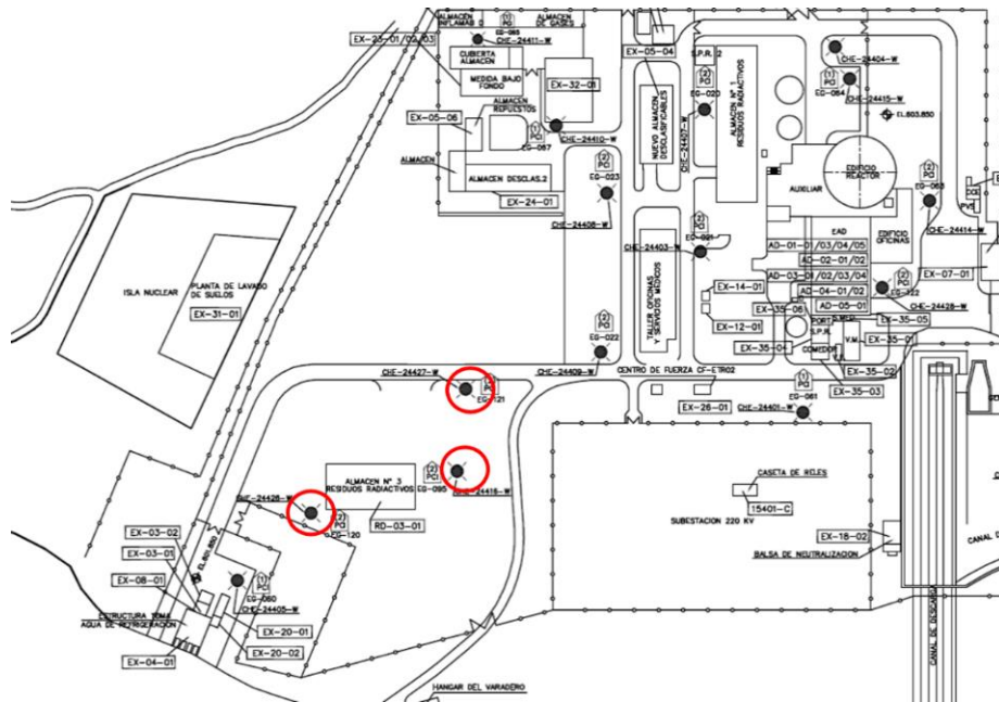
Figura 39. Localización de CHEs a desmantelar
