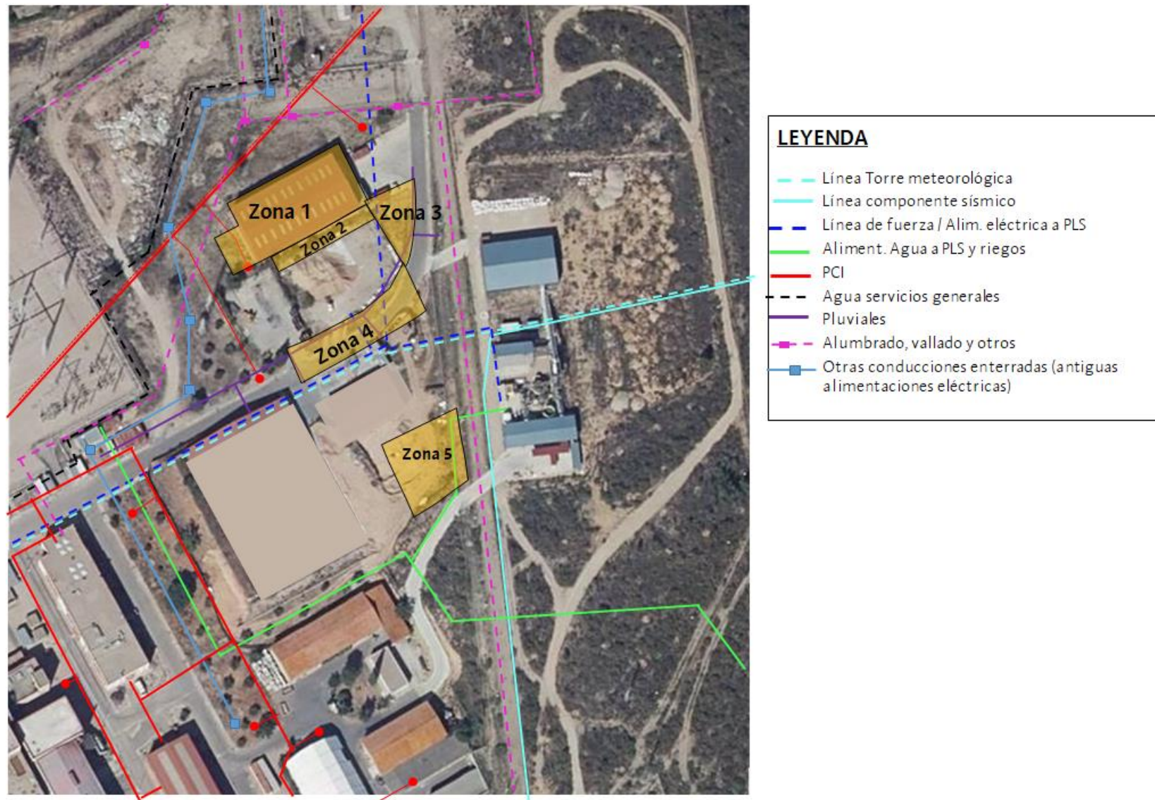
10.- Interferencias. Sistemas afectados
