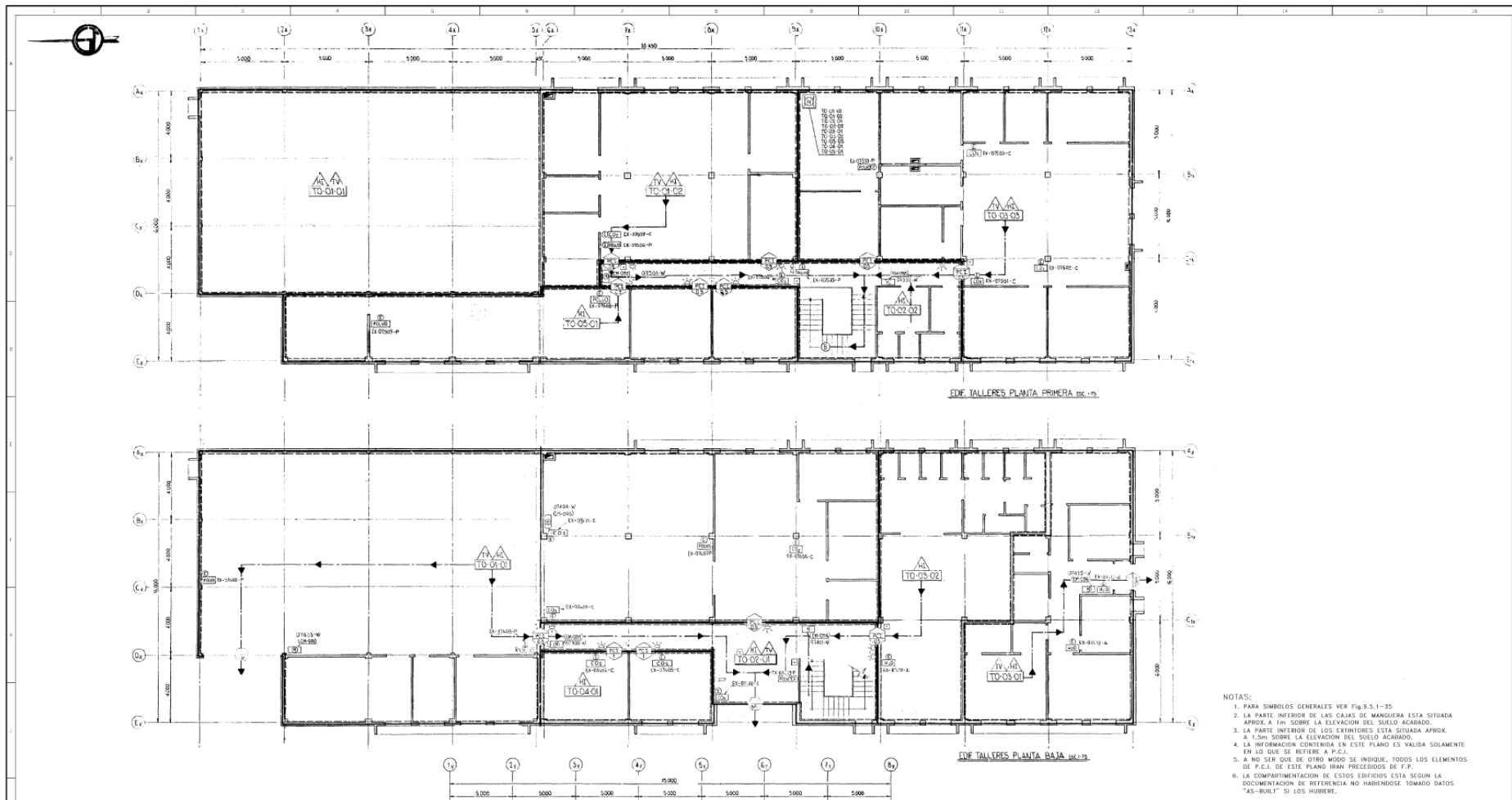
9.- Edificio Oficinas y Talleres. Distribución
