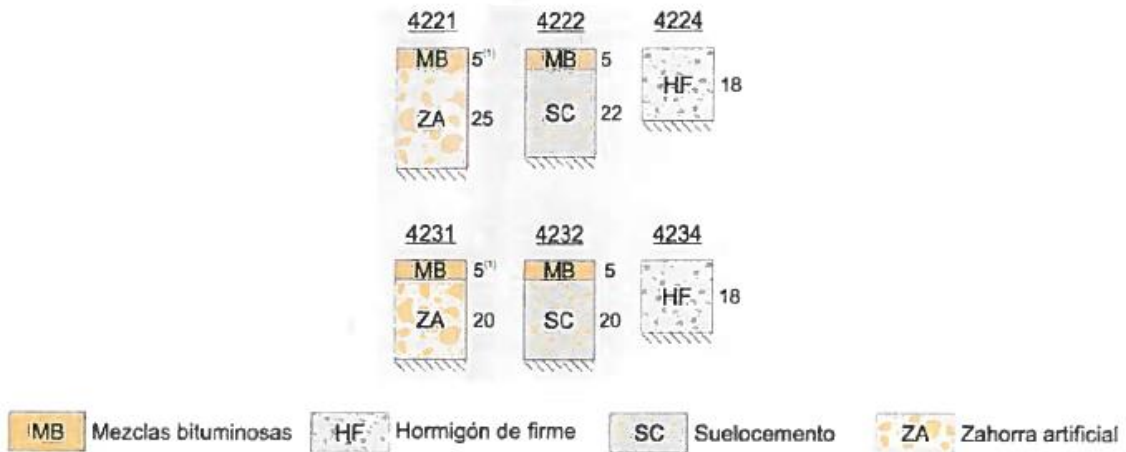
Figura 22 – Tipología de firme
