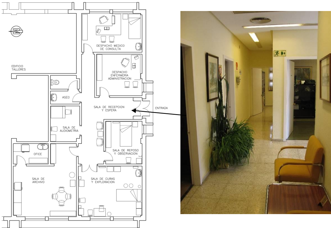
Figura 9. Disposición Servicio Médico
