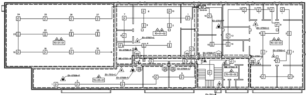
Figura 34 –Disposición del sistema de PCI del edificio de Oficinas y Talleres (El. 607)
