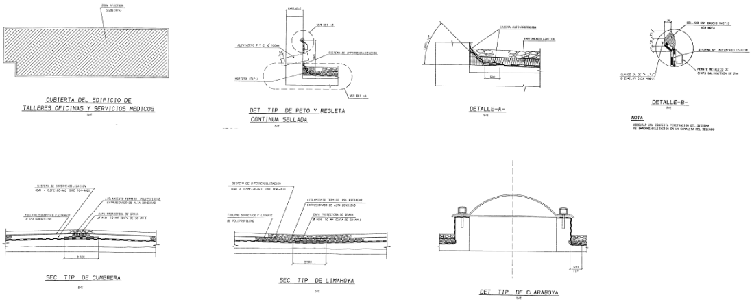
Figura 45. Detalle cubierta oficinas y talleres
