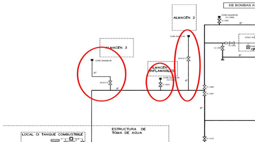
Figura 40. Disposición de ramales de CHEs a desmantelar
