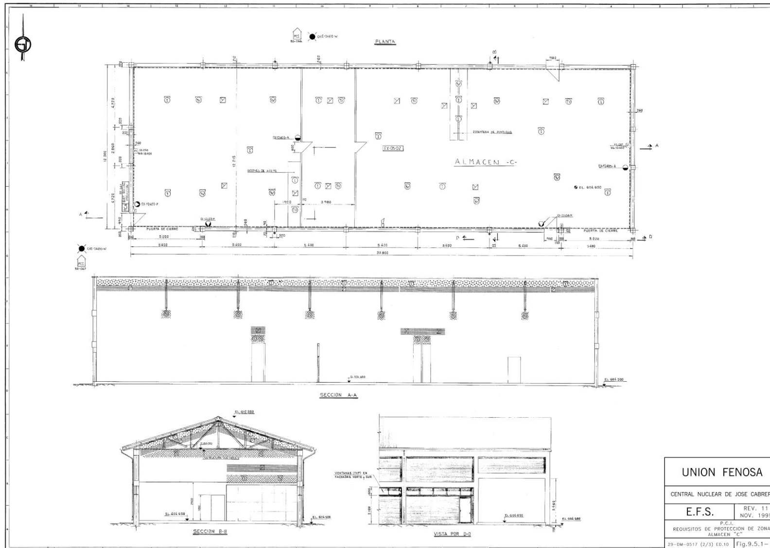
6.- Almacén Desclasificables. Configuración original
