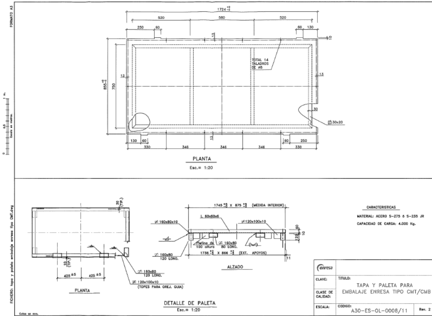
22.- Tapa y paleta embalaje tipo CT/CMB
