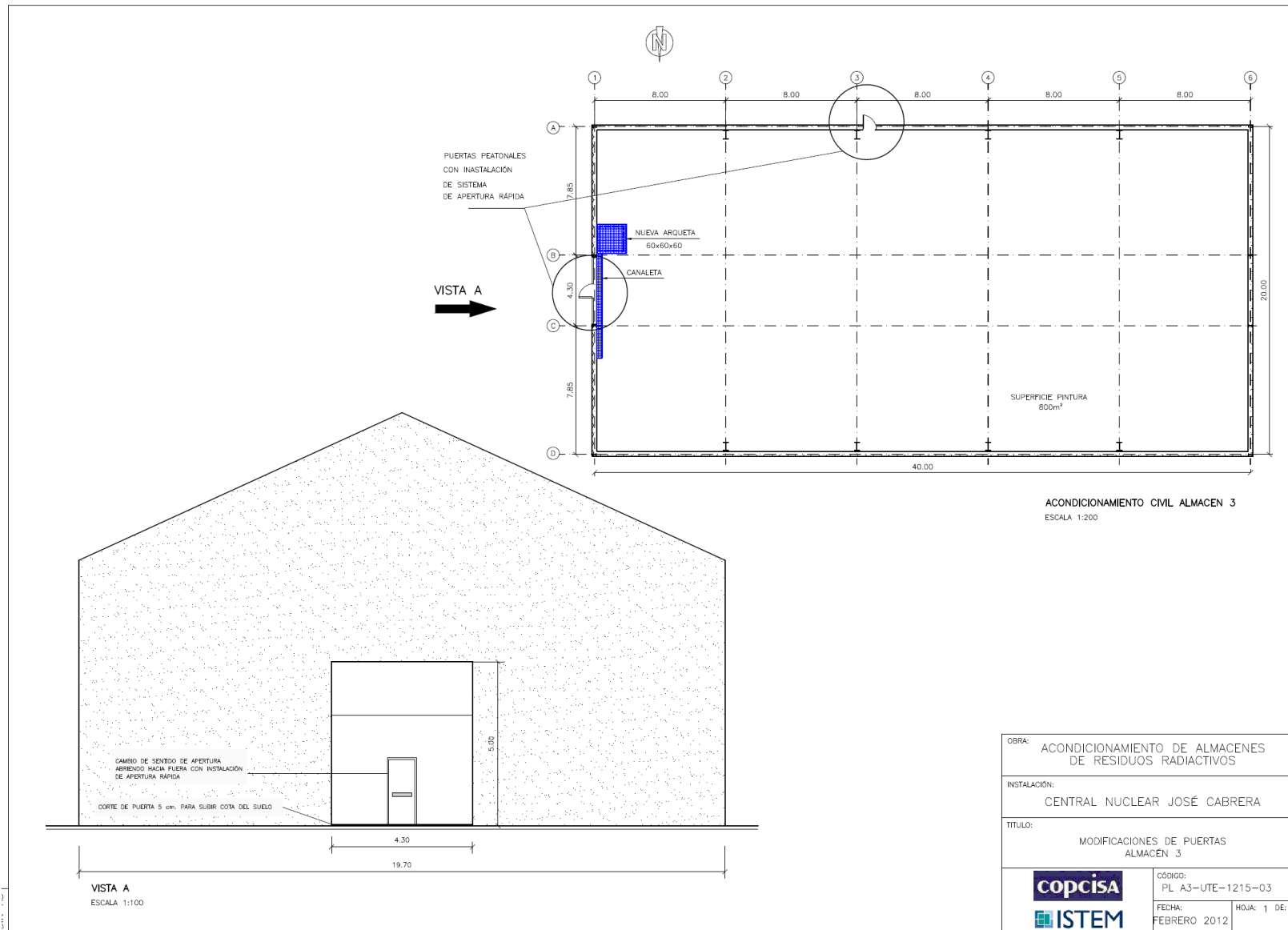
3.- Almacén 3. Alzado y detalle acceso
