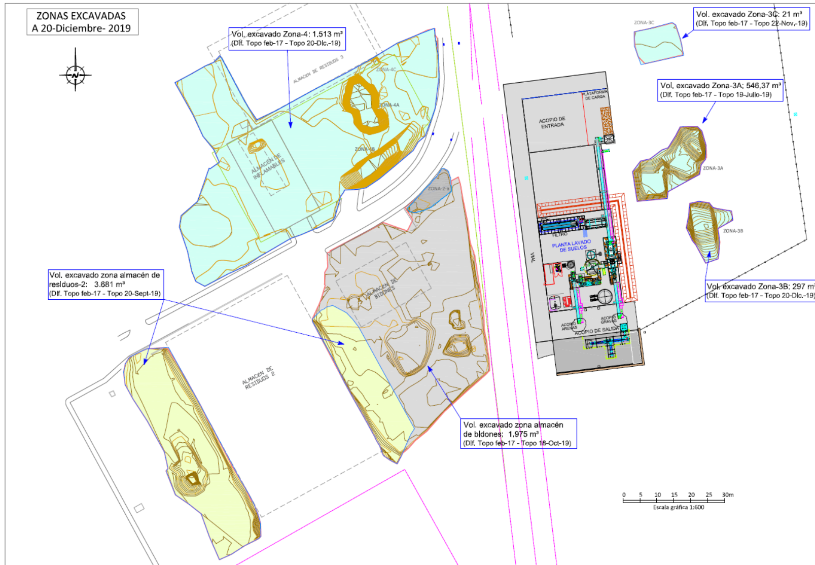
15.- Estado actual de excavaciones en el entorno.
