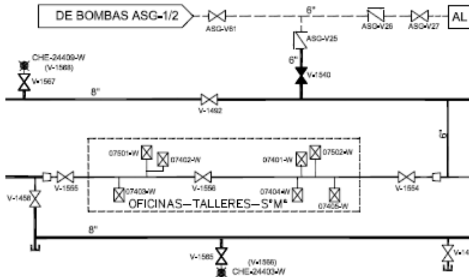
Figura 37 –Esquema de acometidas del anillo de PCI al edificio de Oficinas y Talleres
