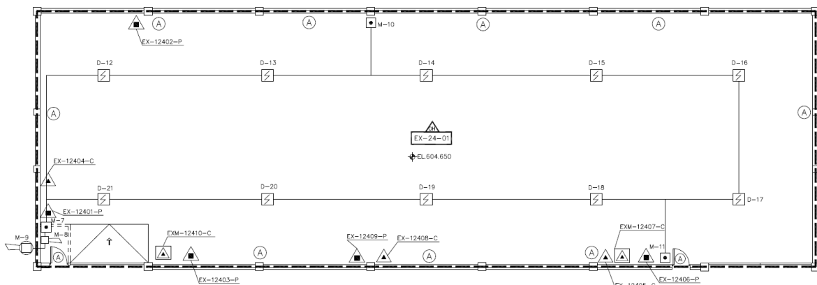
Figura 35 –Disposición del sistema de PCI del almacén de desclasificables
