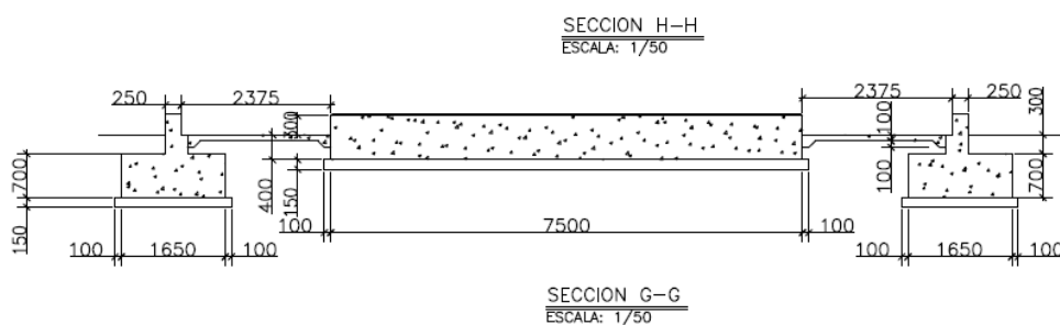
Ilustración 29 Detalle de las Estructuras asociadas al Tanque de Gasoil a demoler
