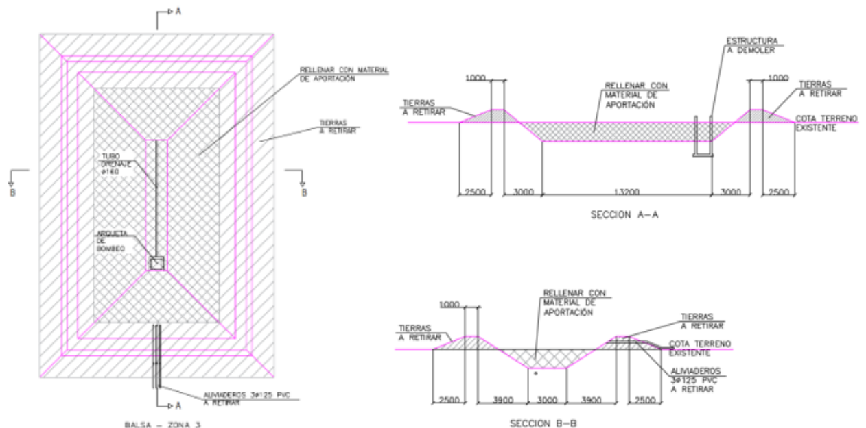
Ilustración 27 Balsa de Decantación
