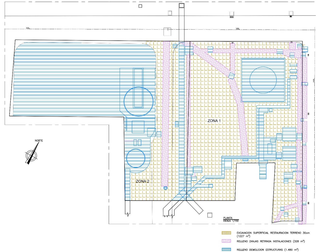
Ilustración 34 Zonas de Excavación
