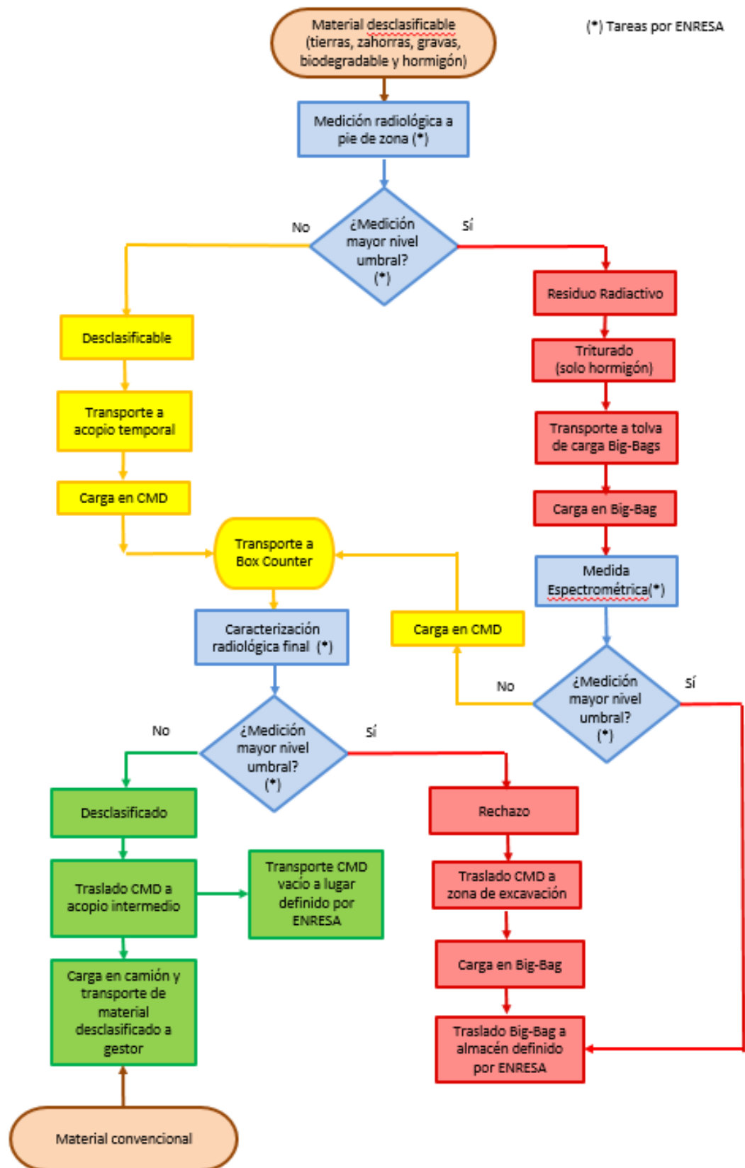
Ilustración 7 Diagrama de Bloques Gestión de Materiales
