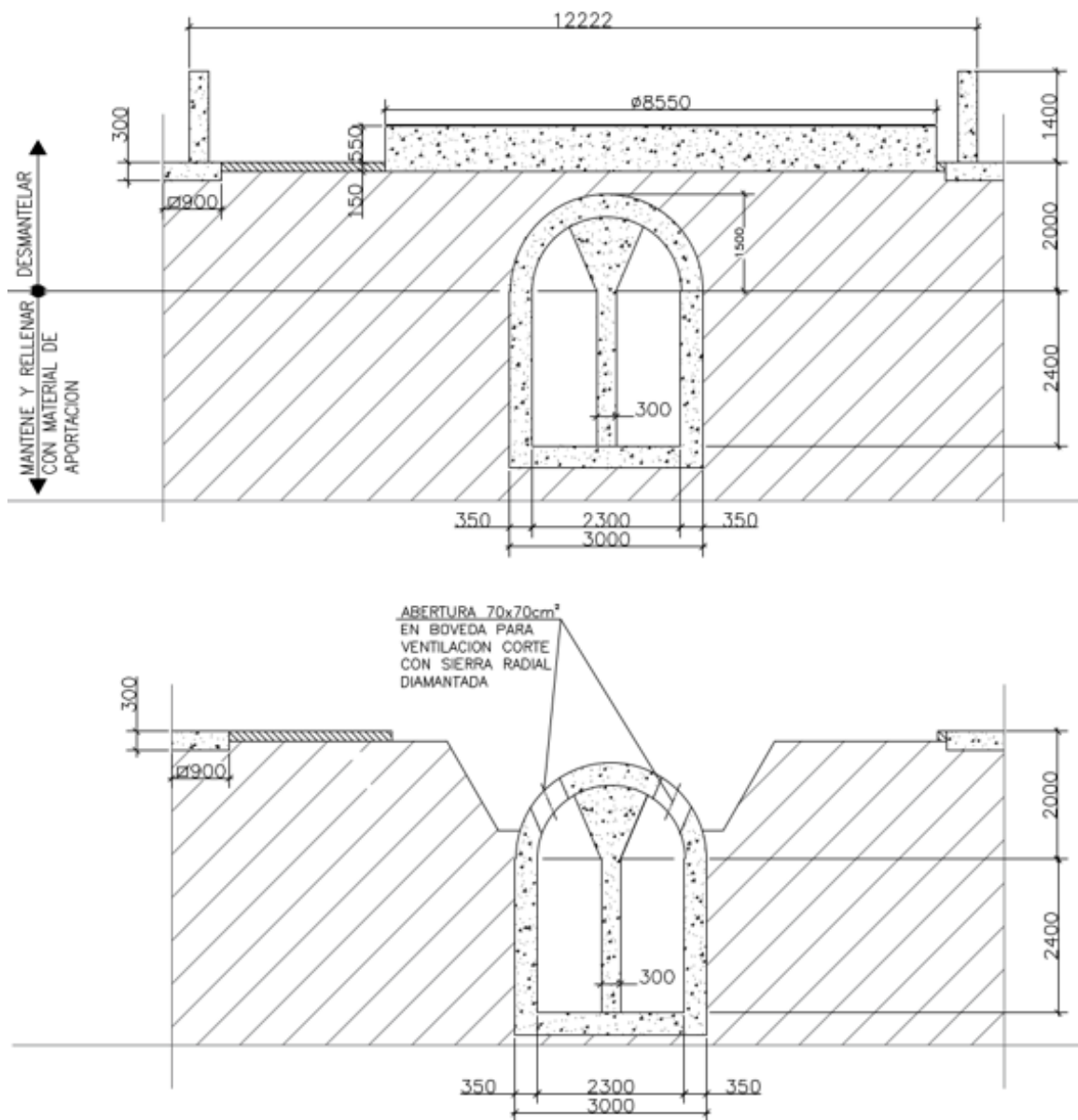
Ilustración 26 Galería de Aceite bajo el Cubeto y el Depósito FH-20*
