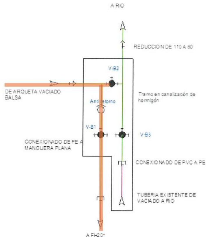
Ilustración 21 Configuración Entronque (en naranja a retirar)
