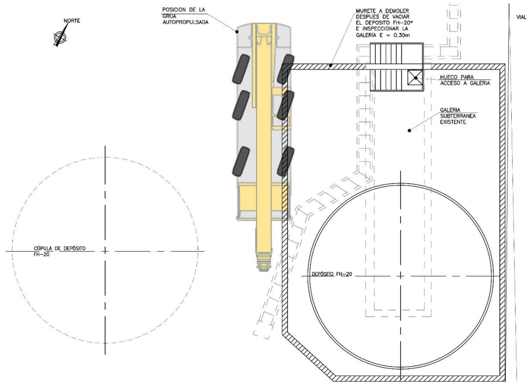
Ilustración 24 Posición de la Grúa Autopropulsada para Retirar la Cúpula
