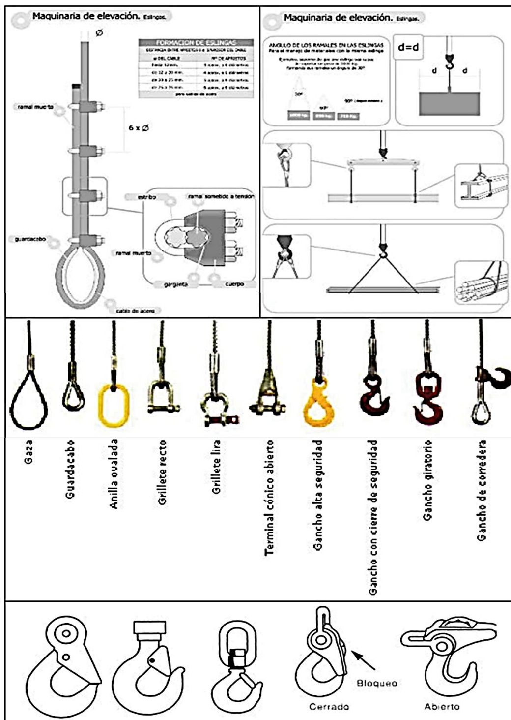
Figura G.20 – Elementos de Elevación I
