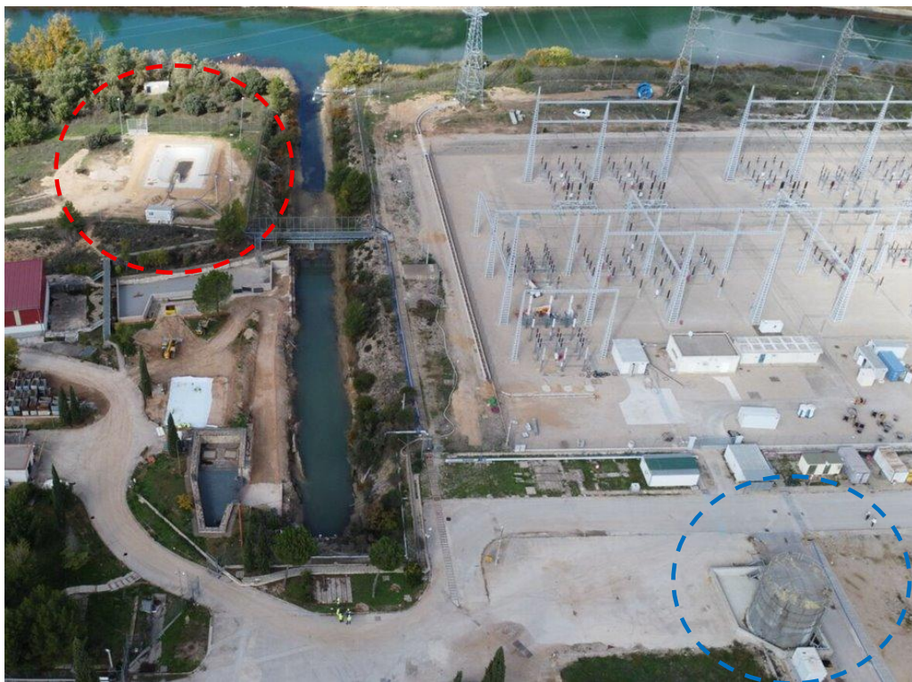
Ilustración 3 Ubicación del Sistema de Tratamiento de Efluentes Líquidos FH20* (azul) y Zona de Balsa de Decantación (rojo)
