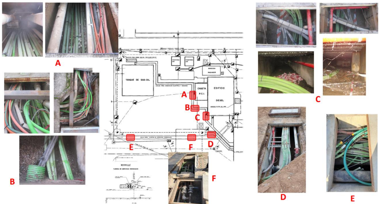
Ilustración 10 Conducciones Eléctricas en Desuso en Zanjas Registrables
