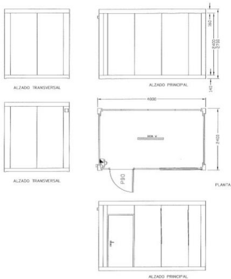
Ilustración 17 Caseta Modular Puesto de Control Radiológico Ro-18
