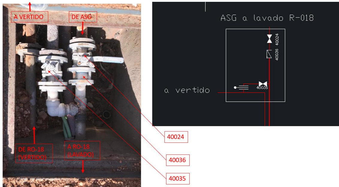
Ilustración 16 Arqueta Conexión Vertido Efluentes Líquidos y Control Radiológico
