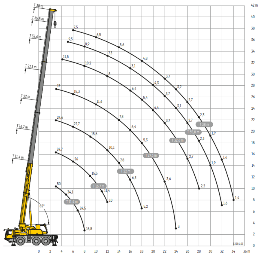
Ilustración 25 Alturas de Elevación de la Grúa Autopropulsada de 50 t
