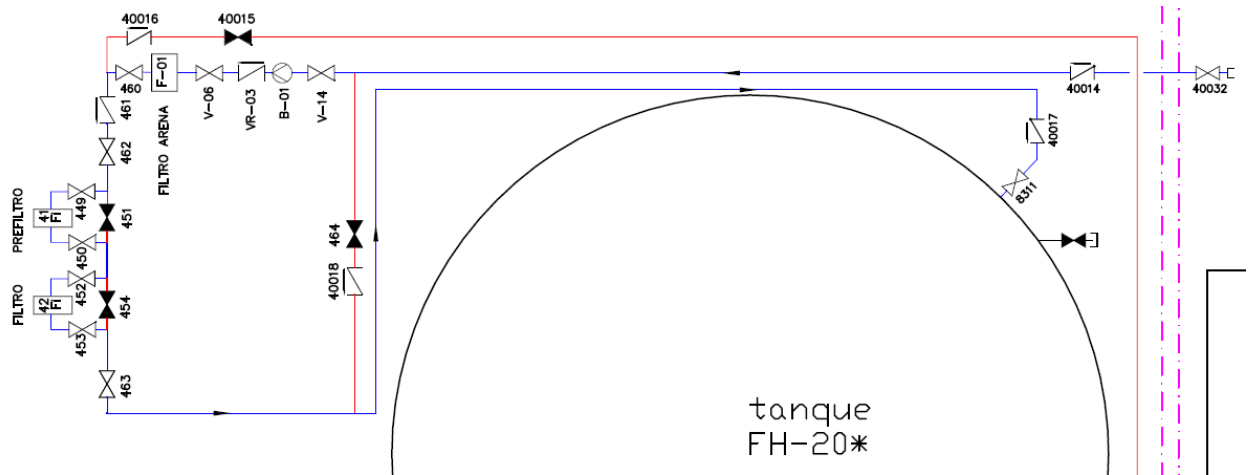
Ilustración 13 Sistema de Tratamiento de Efluentes Líquidos
