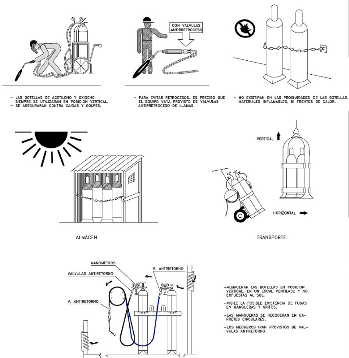
Figura G.16 – Trabajos con Oxiacetileno
