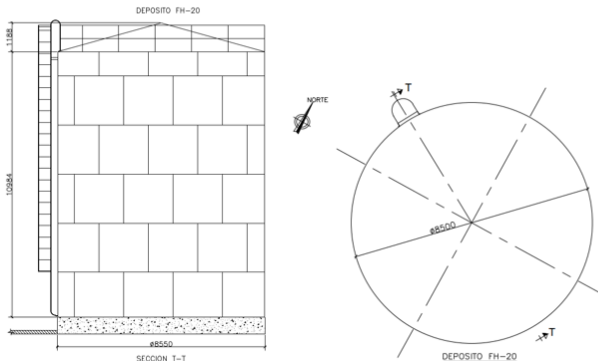
Ilustración 23 Depósito FH-20* (Alzado y Planta)
