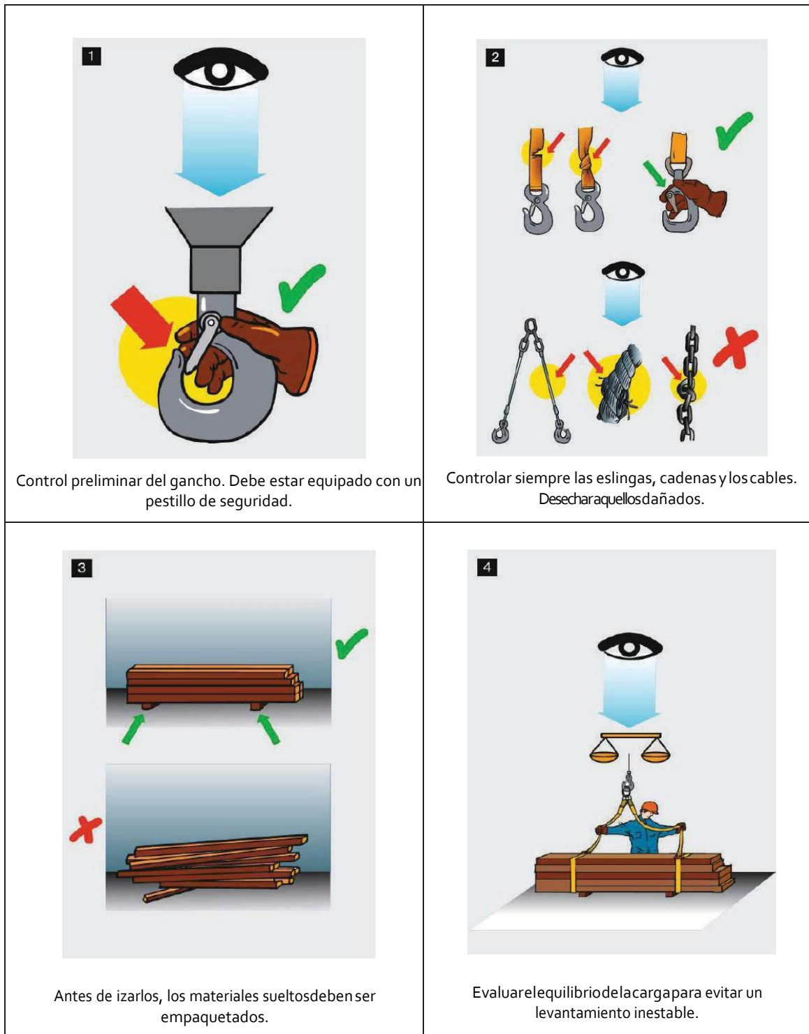
Figura G.17 – Izado de Cargas 1
