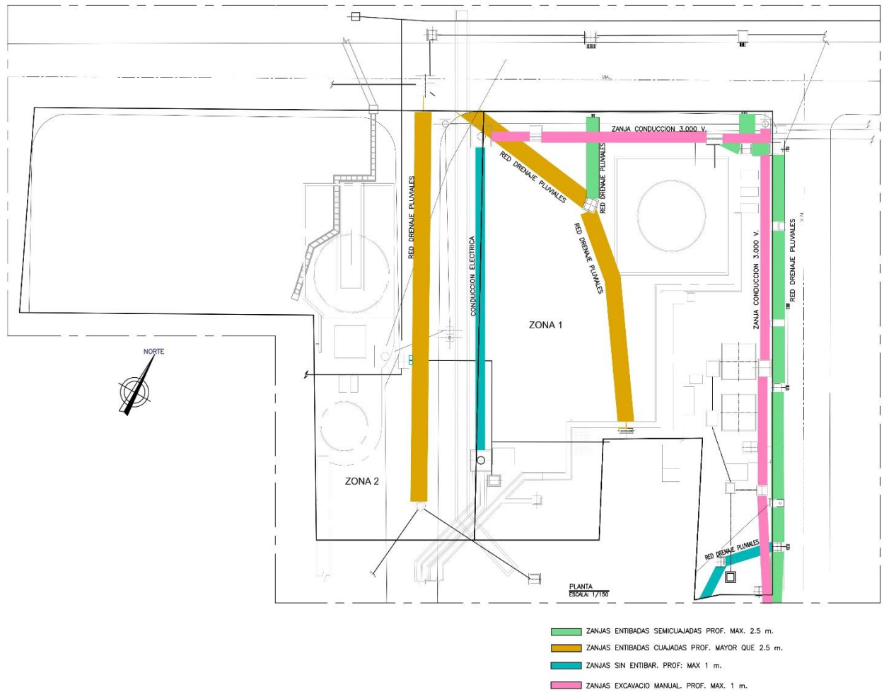
Ilustración 11 Zanjas para Retirada de Conducciones a Retirar o para Protección de Conducciones a Mantener
