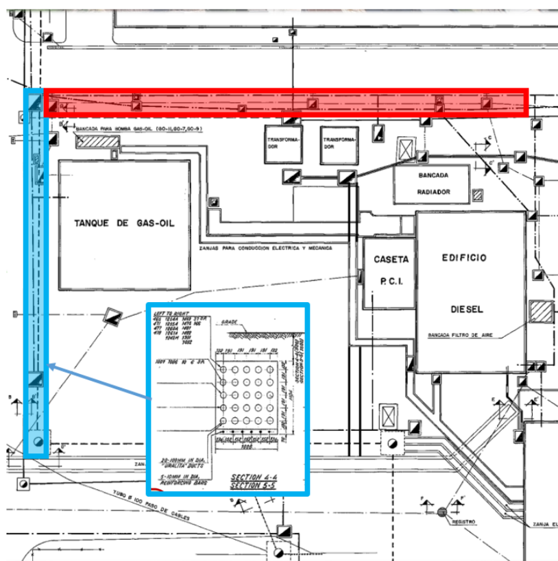
Ilustración 32 Zonas de Canalizaciones Eléctricas en Servicio
