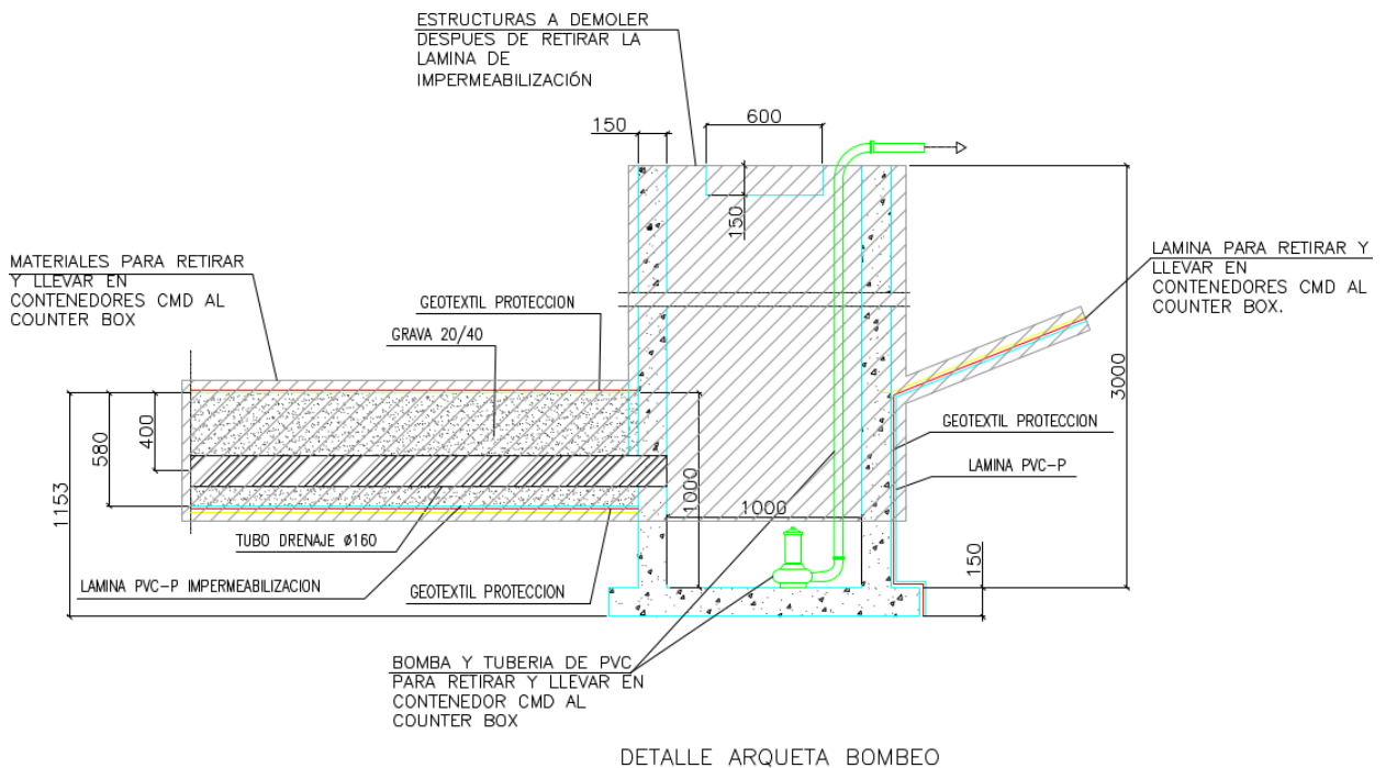
Ilustración 28 Detalles de la Balsa de Decantación
