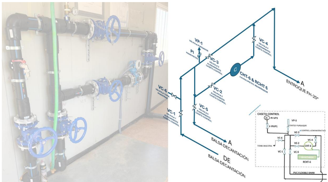
Ilustración 22 Colector Mural Interior Puesto de Control
