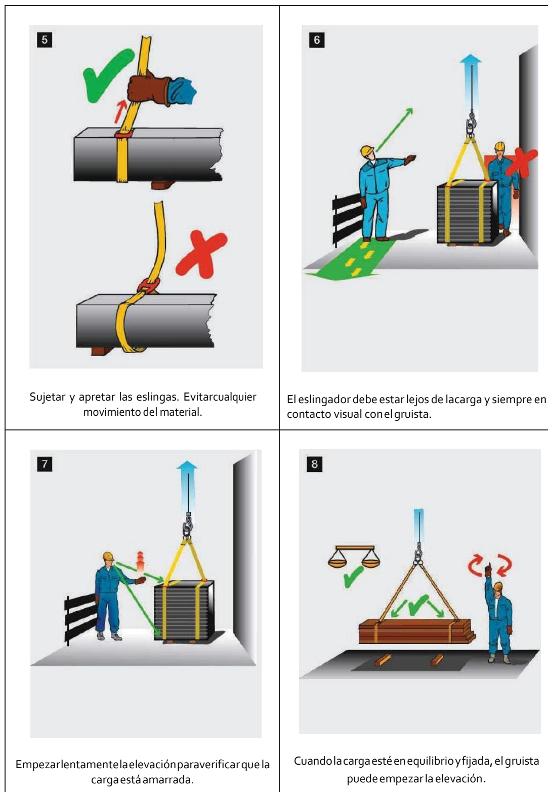
Figura G.18 – Izado de Cargas 2
