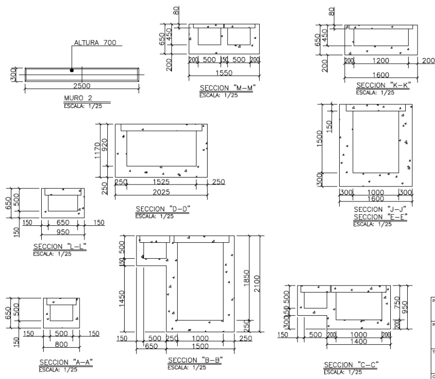
Ilustración 30 Detalles de las Zanjas Registrables a demoler
