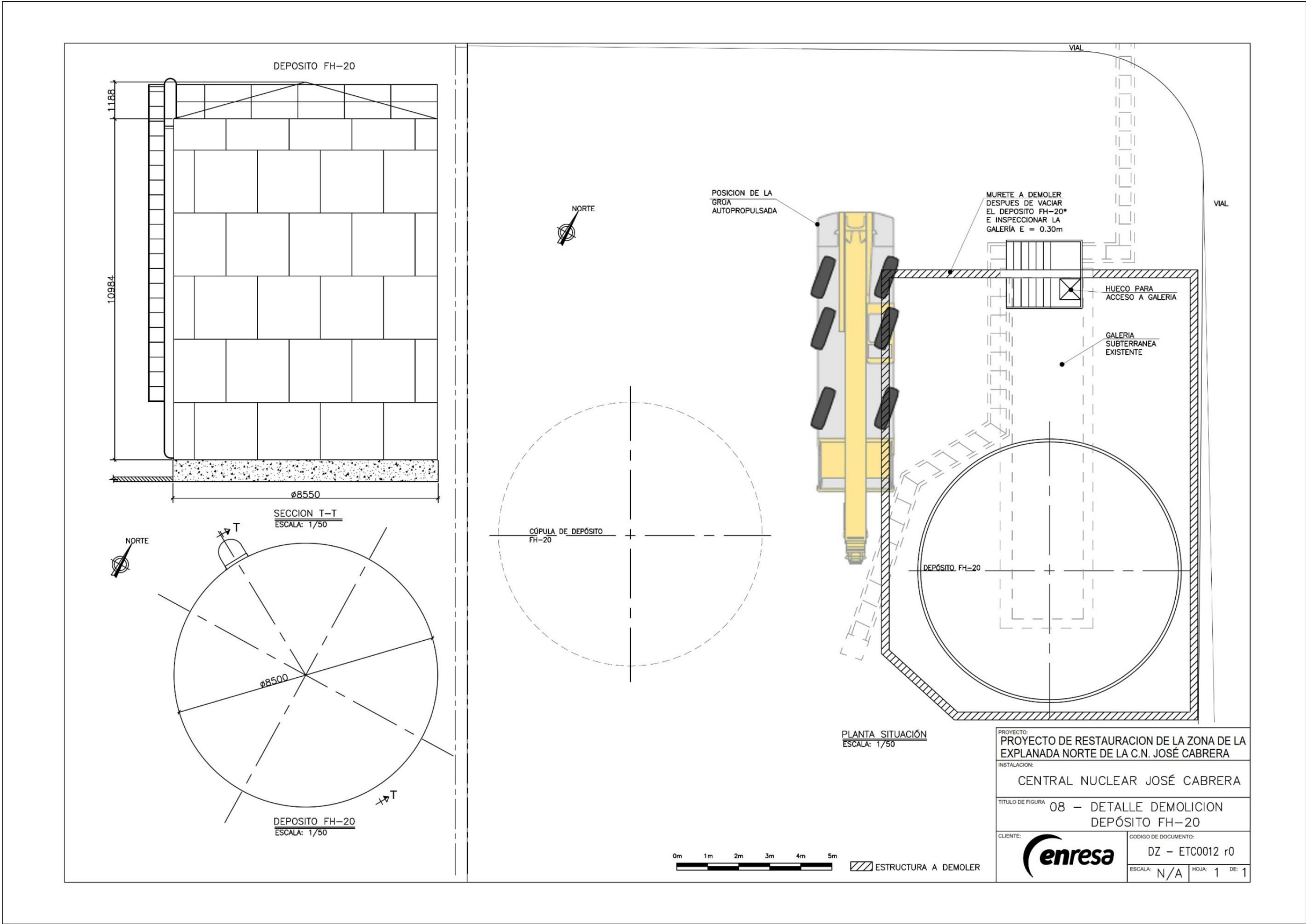
Figura B.8 Detalle Demolição Depósito FH-20*
